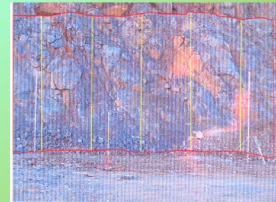
Beispiel für eine Vermessene Wand mit eingezeichneten Bohrlöchern und aufgestellten Meßlatzen Gelbe Linien: Beispiele für Bohrlöcher (Sollvorgabe) Rote Linie: Begrenzung der Meßfläche (Sprengbereich)
